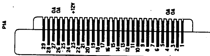
Brochage du connecteur (alimentation 12V)
